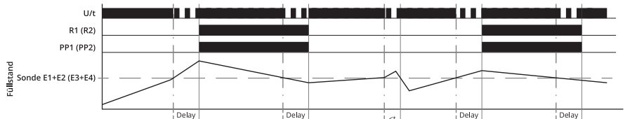
Při použití jedné sondy v nádrži
