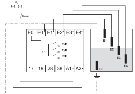
Schéma zapojení
