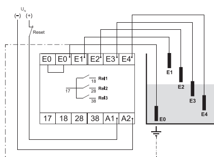
Schéma zapojení
