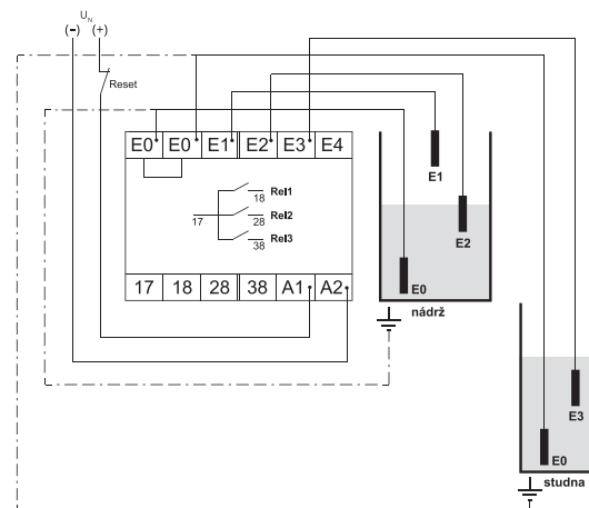
Schéma zapojení
