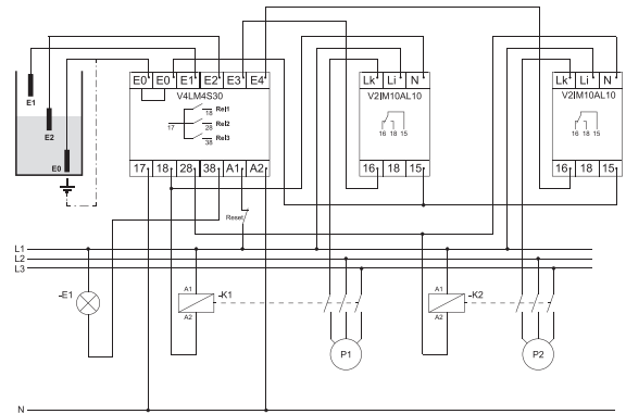
Schéma zapojení
