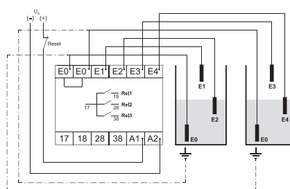
Schéma zapojení s oddělenými sondami
